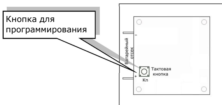
Рисунок 6.4. Плата радиокнопки вызова MP-411D1
