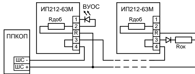
Рис.2 Типовая схема включения извещателя для приборов с переполюсовкой шлейфа сигнализации. Величина резисторов Rok и Rдоб определяется в соответствии с техническим описанием ППКОП
