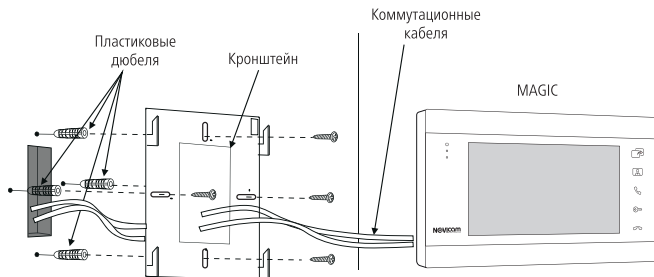
Рис. 4 Монтаж видеодомофона
