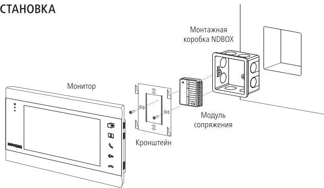
Рис. 4 Монтаж видеодомофона
