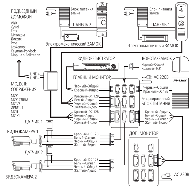
Рис. 7 Схема подключения видеодомофонов MAGIC HD
