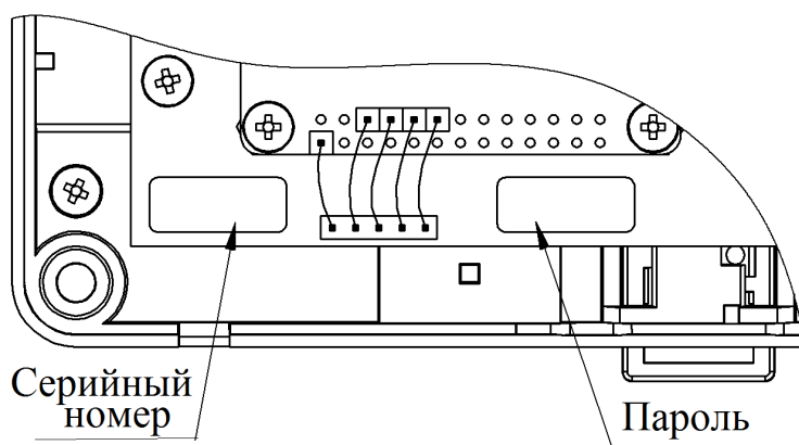
Рис.8 Расположение наклеек УС.
