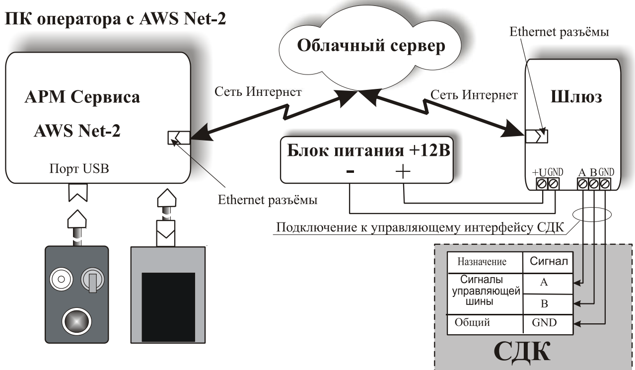
Рис.3 Схема подключения УС (Шлюза) к облачному ССДК
