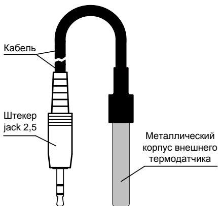
Рис.4 Внешний термодатчик
