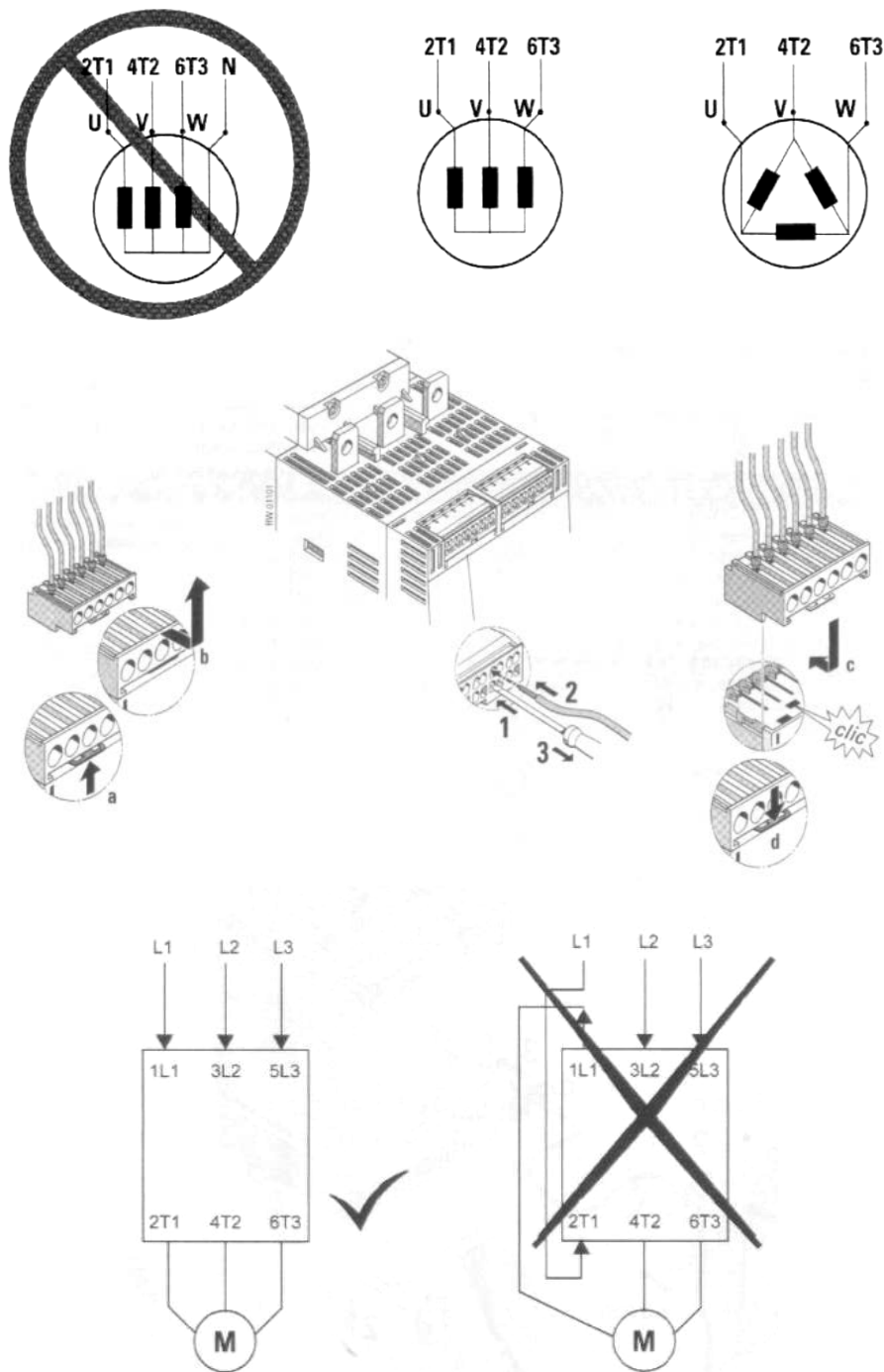
Рисунок 11. Схема подключения без нейтрали.
