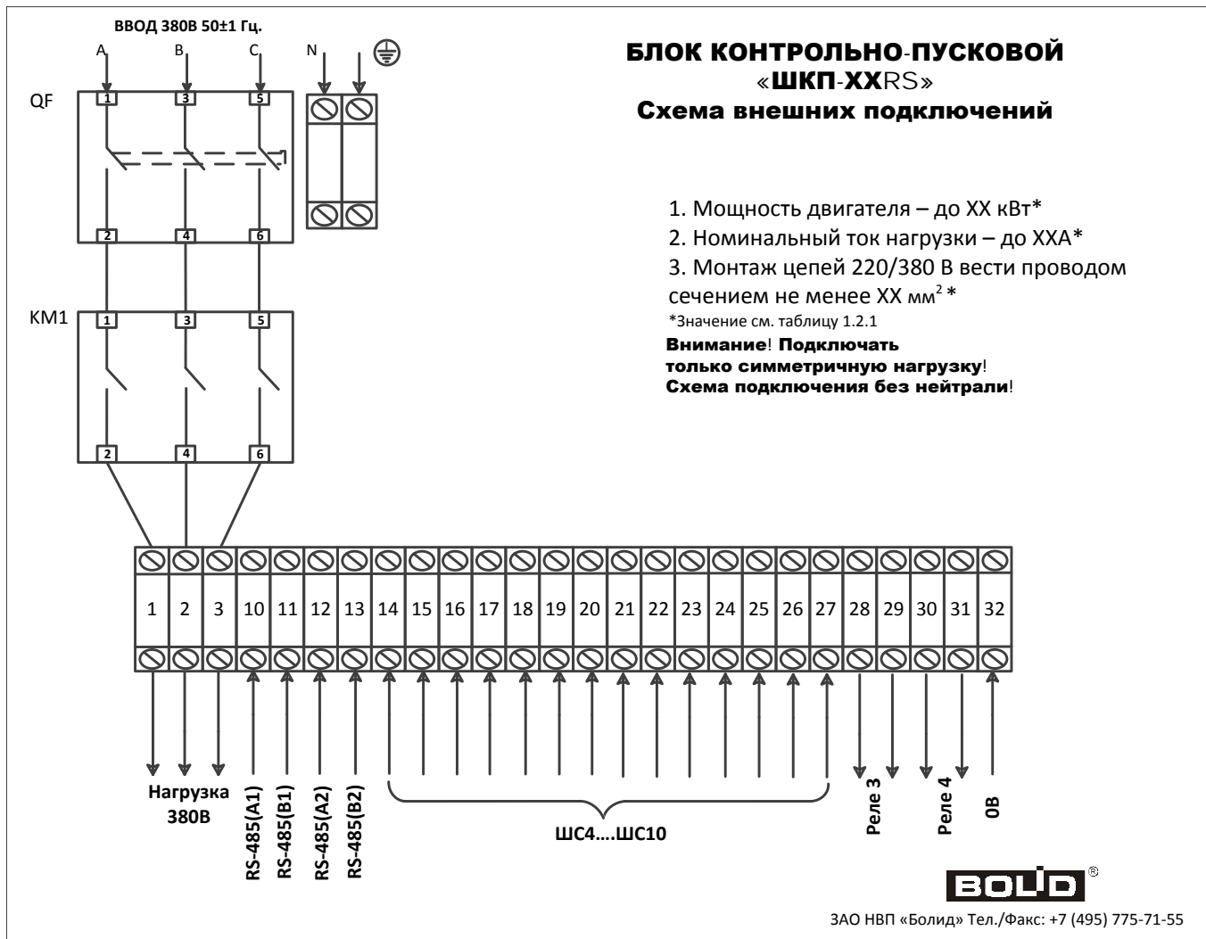
Рисунок 3а. Схема подключения блоков ШКП-XXRS при 380В.
