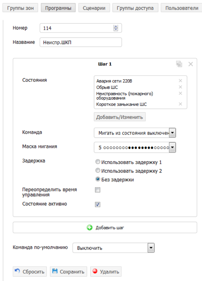
Рисунок 8. Настройка шага программы управления индикатора «неисправность».
