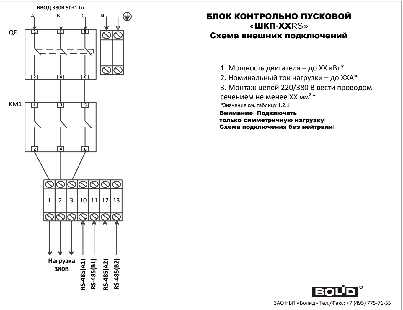
Рисунок 36. Схема подключения блоков ШКП-XXRS (М) при 380В.
