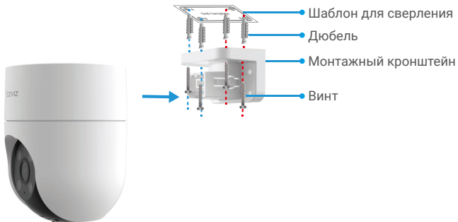
Рисунок 1. Монтаж на потолок
