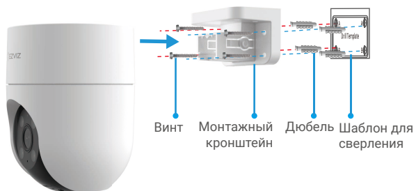
Рисунок 2. Монтаж на стену
