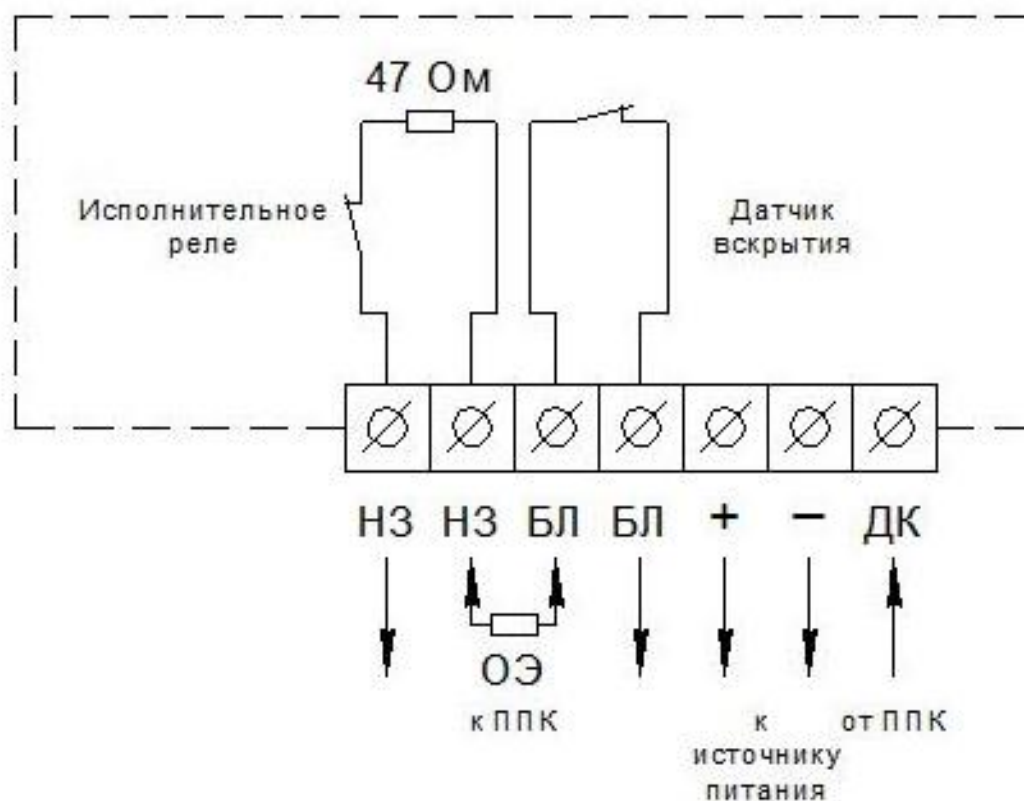
Рисунок 2.6 – Колодка извещателя для внешних подключений
