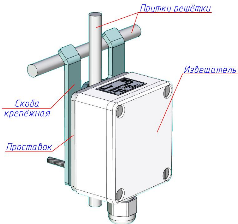
Рисунок 2.1 – Крепление извещателя на решетке из прутка
