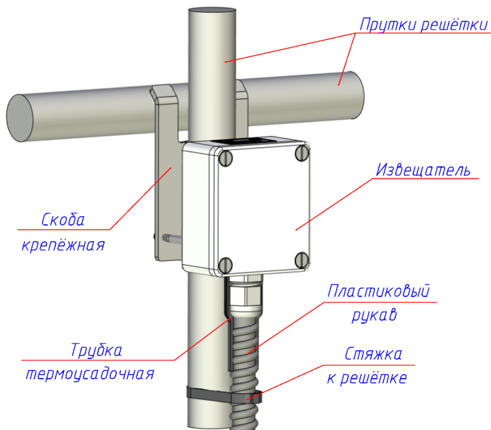
Рисунок 2.7 – Крепление кабеля извещателя
