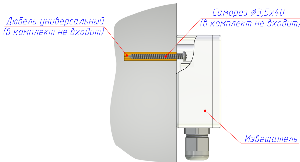
Рисунок 2.5 – Крепление извещателя
