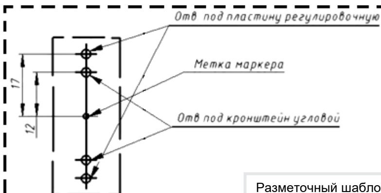
Разметочный шаблон
