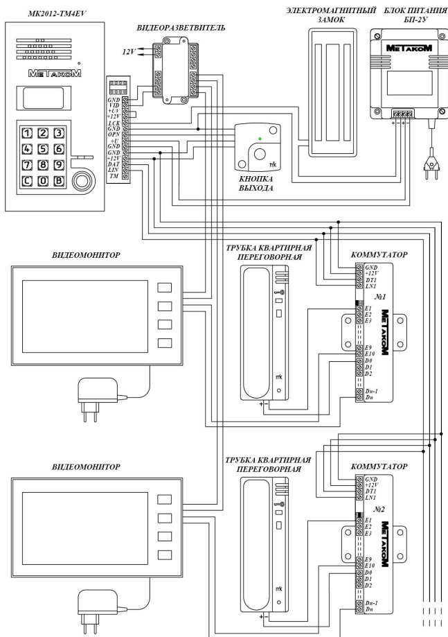
Рис. 3 Пример монтажа блока вызова МК2012-ТМ4ЕУ при использовании нескольких коммутаторов.
