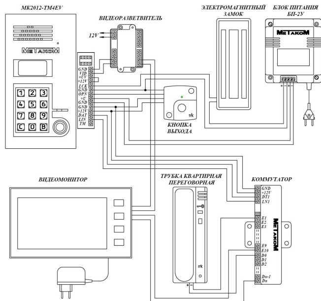
Рис. 2 Пример монтажа блока вызова МК2012-TM4EV
