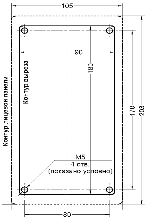
Рис. 1 Разметка под установку блока вызова
