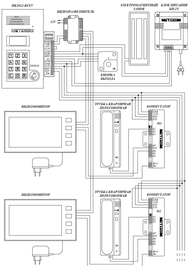
Рис. 3 Пример монтажа блока вызова МК2012-RF(MF)EV при использовании нескольких коммутаторов.
