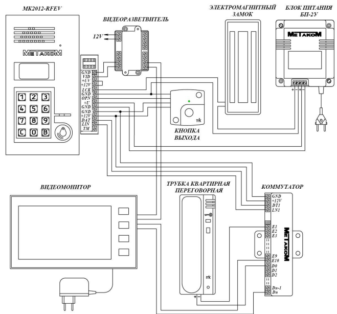
Рис. 2 Пример монтажа блока вызова МК2012-RF(MF)EV
