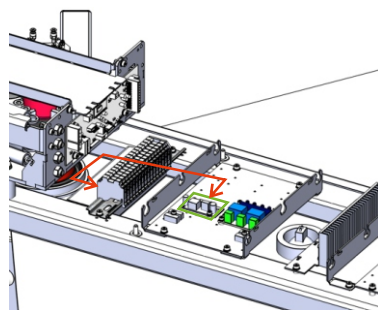
Клеммная колодка
