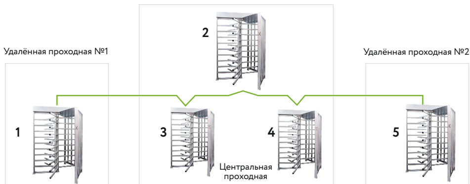
Рисунок 9.27 - Пример размещения оборудования
