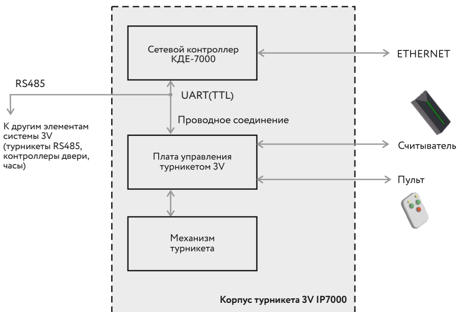
Рисунок 2.3 – Структура турникета IP7000
