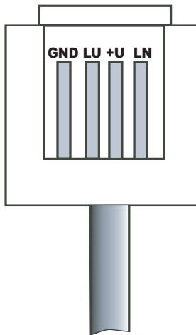
Рис.3 Порядок расположения линий ПК на разъеме шнура SCO-1-6P4C
