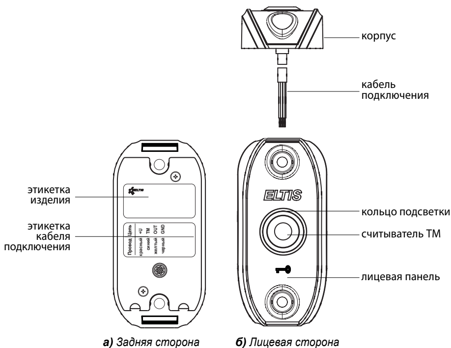
Рис.1 Внешний вид блока электронного ключевого устройства CRT-71
