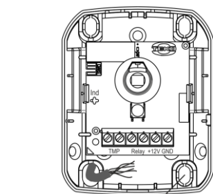
Заглушка отверстия для проводов
