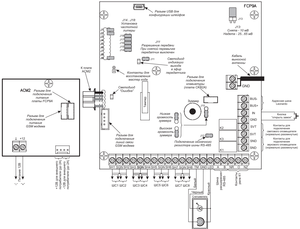
Рис. 13. Монтажная схема прибора
