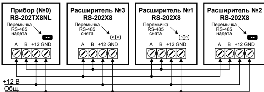
Рис. 12. Пример подключения расширителей к прибору.
