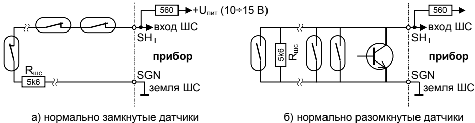
Рис. 8. Примеры монтажа охранных шлейфов
