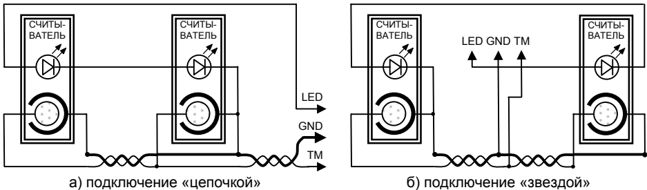
Рис. 10. Подключение двух считывателей
