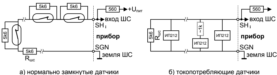
Рис. 9. Примеры монтажа пожарных шлейфов
