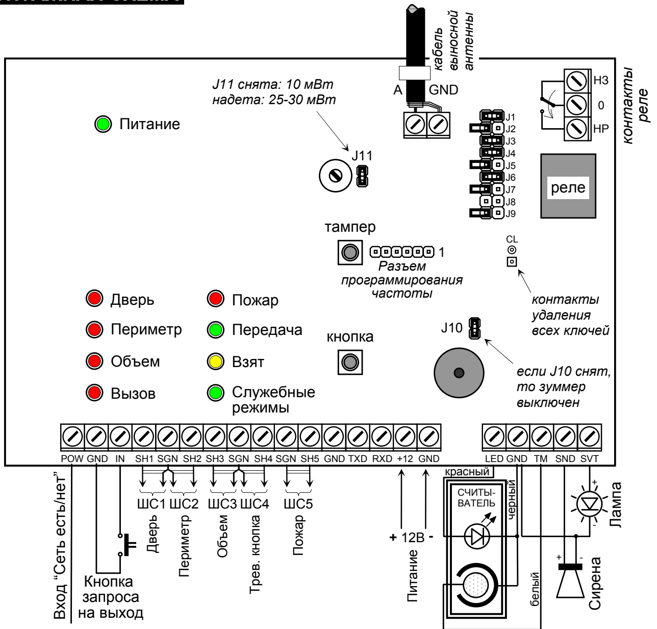
Рис. 7. Монтажная схема передатчика
