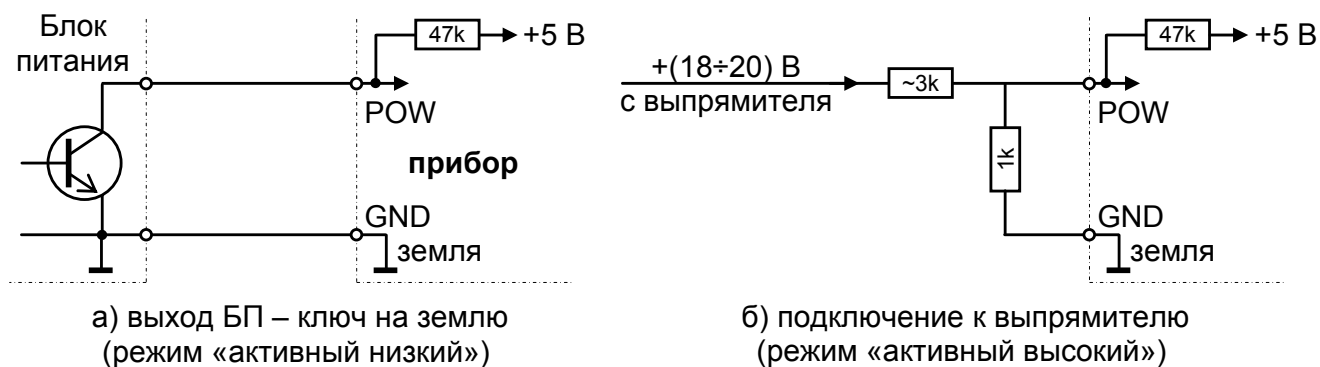
Рис. 4. Примеры монтажа входа POW (контроль сети 220 В)
