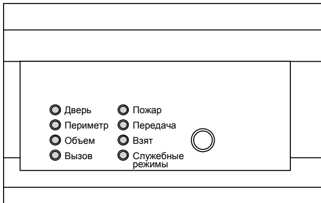
Рис. 1. Внешний вид передатчика
