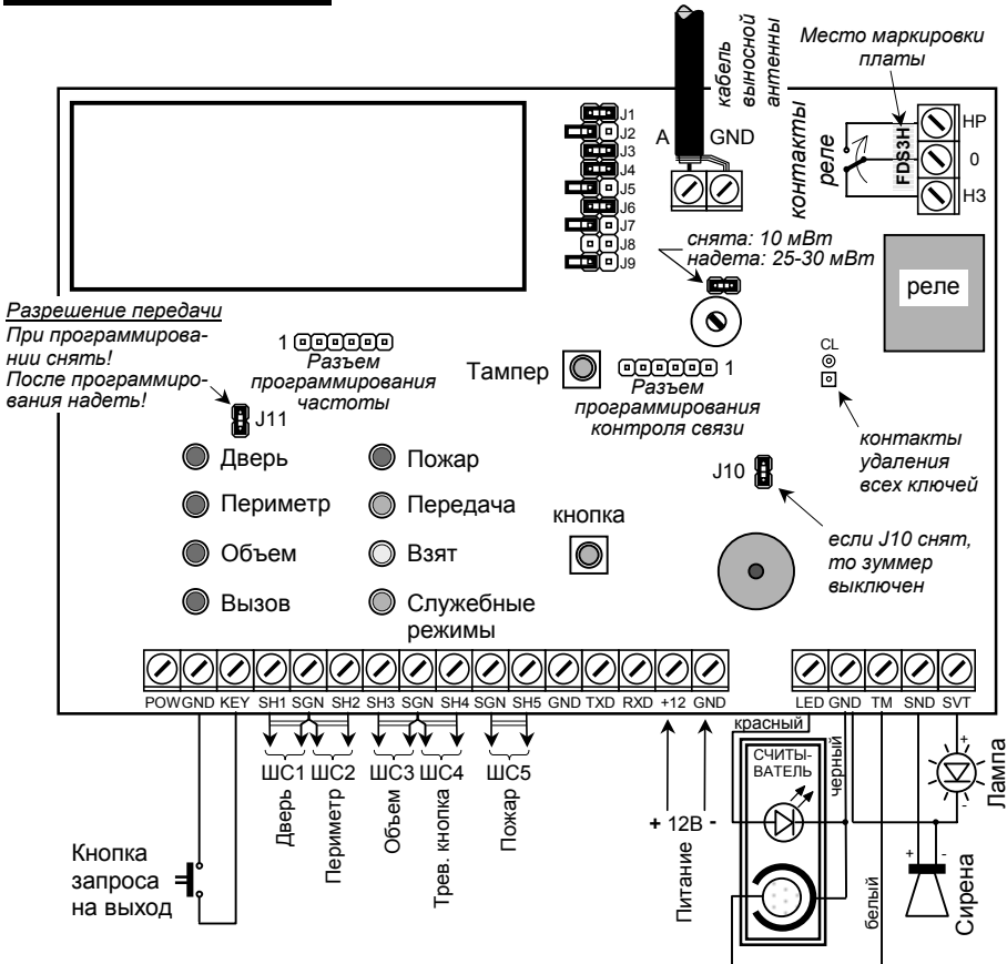
Рис. 7. Монтажная схема передатчика
