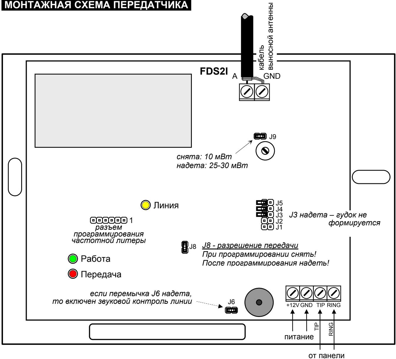
Рис. 2. Монтажная схема передатчика
