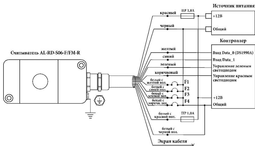
Рисунок 4 – Схема подключения считывателя AL-RD-S06-F/FM-R к контроллеру СКУД с разделным питанием считывателя и нагревателя.
