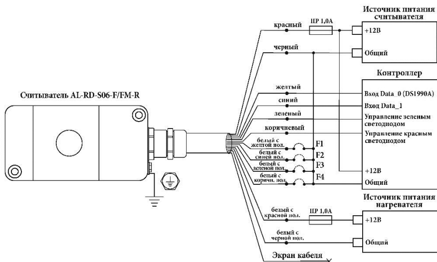
Рисунок 4 – Схема подключения считывателя AL-RD-S06-F/FM-R к контроллеру СКУД с разделным питанием считывателя и нагревателя.
