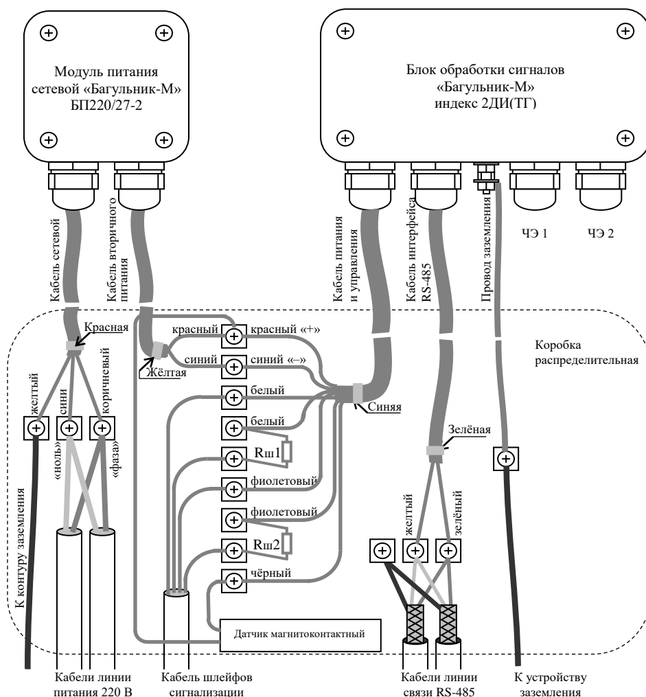
Рис. 8.9. Общий пример подключения изделия «Багульник-М»
