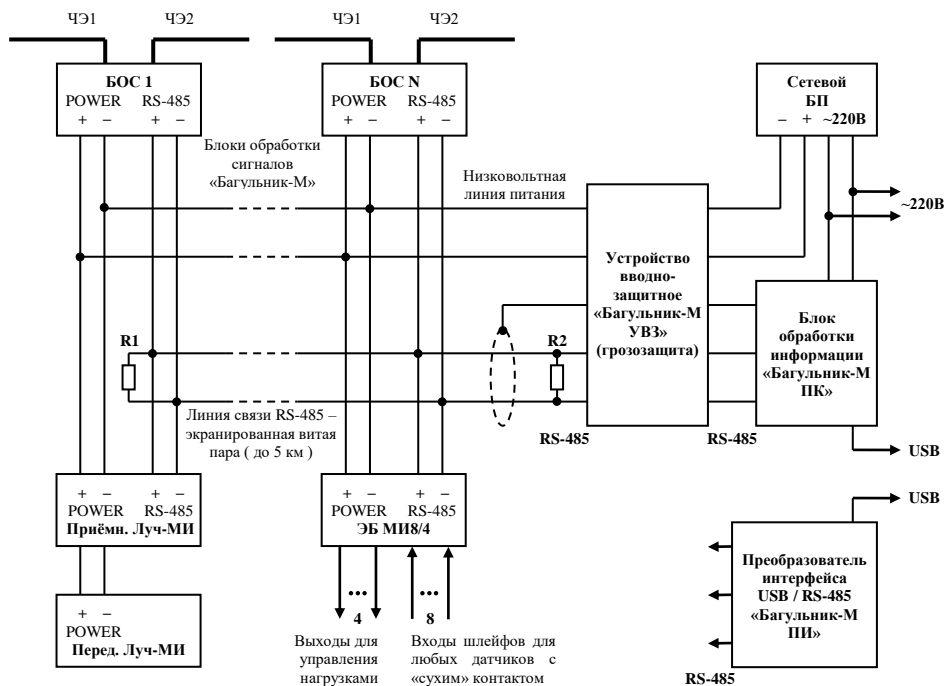
Рис. 8.12. Вариант построения системы сбора информации по интерфейсу RS-485
