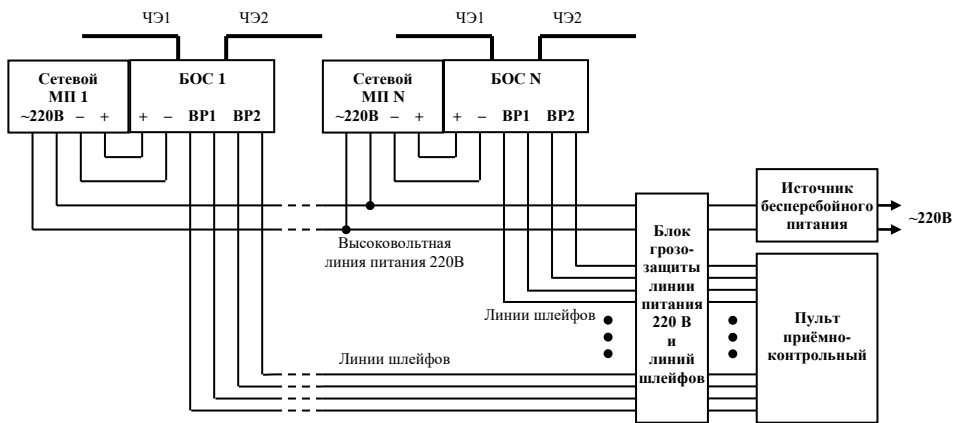
Рис. 8.11. Система сбора со шлейфами сигнализации с питанием от линии 220 В
