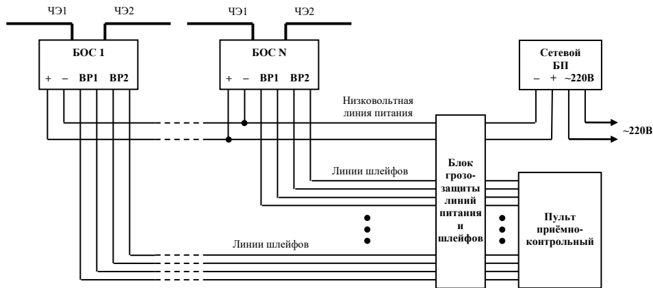
Рис. 8.10. Система сбора со шлейфами сигнализации и низковольтным питанием
