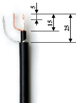
Рис. 8.3. Образец разделки кабелей ЧЭ для подключения к БОС
