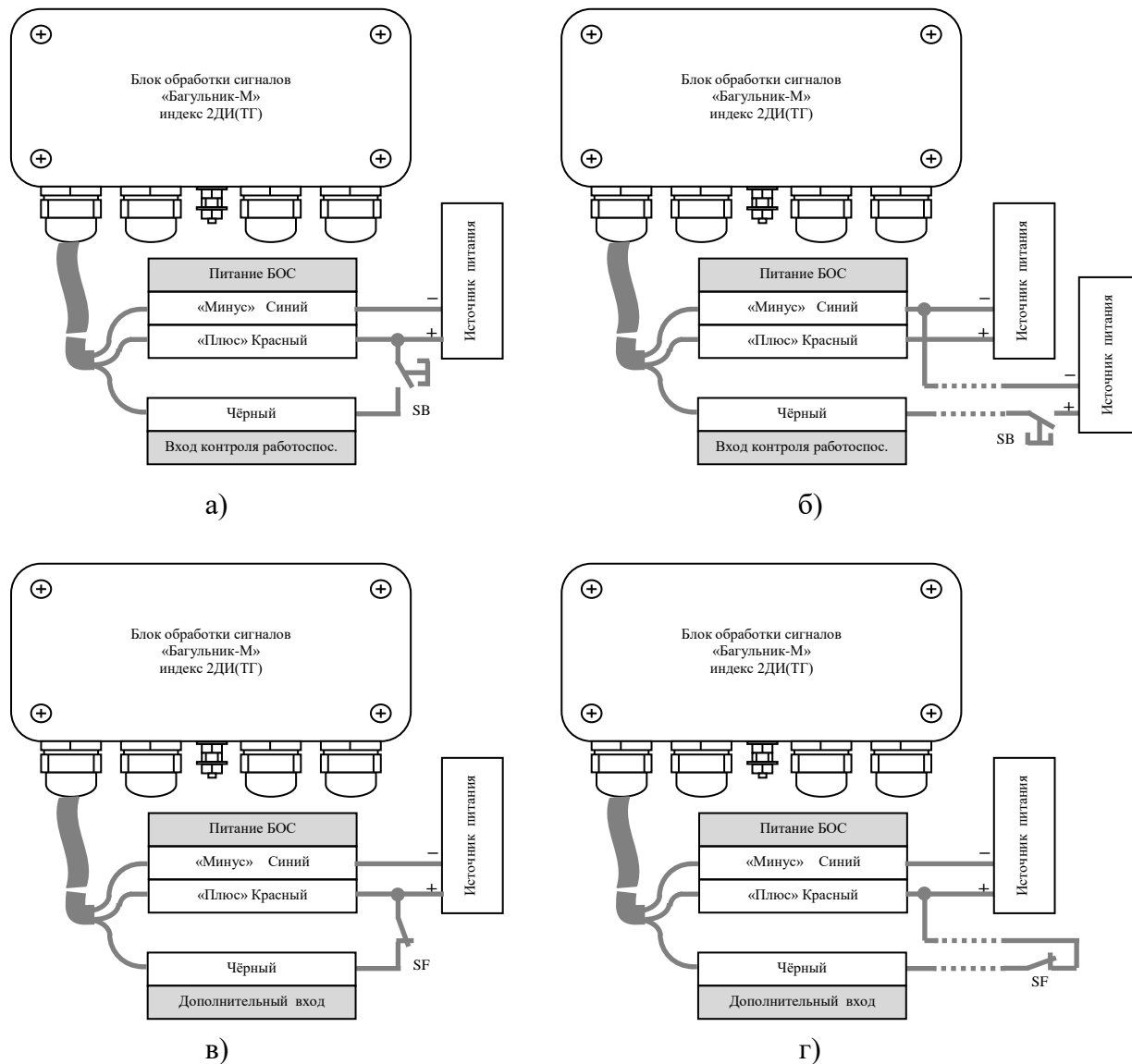
Рисунок 8.8. Подключение входа контроля работоспособности/доп. входа
