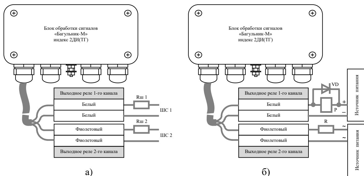
Рисунок 8.6. Примеры подключения выходных реле изделия
