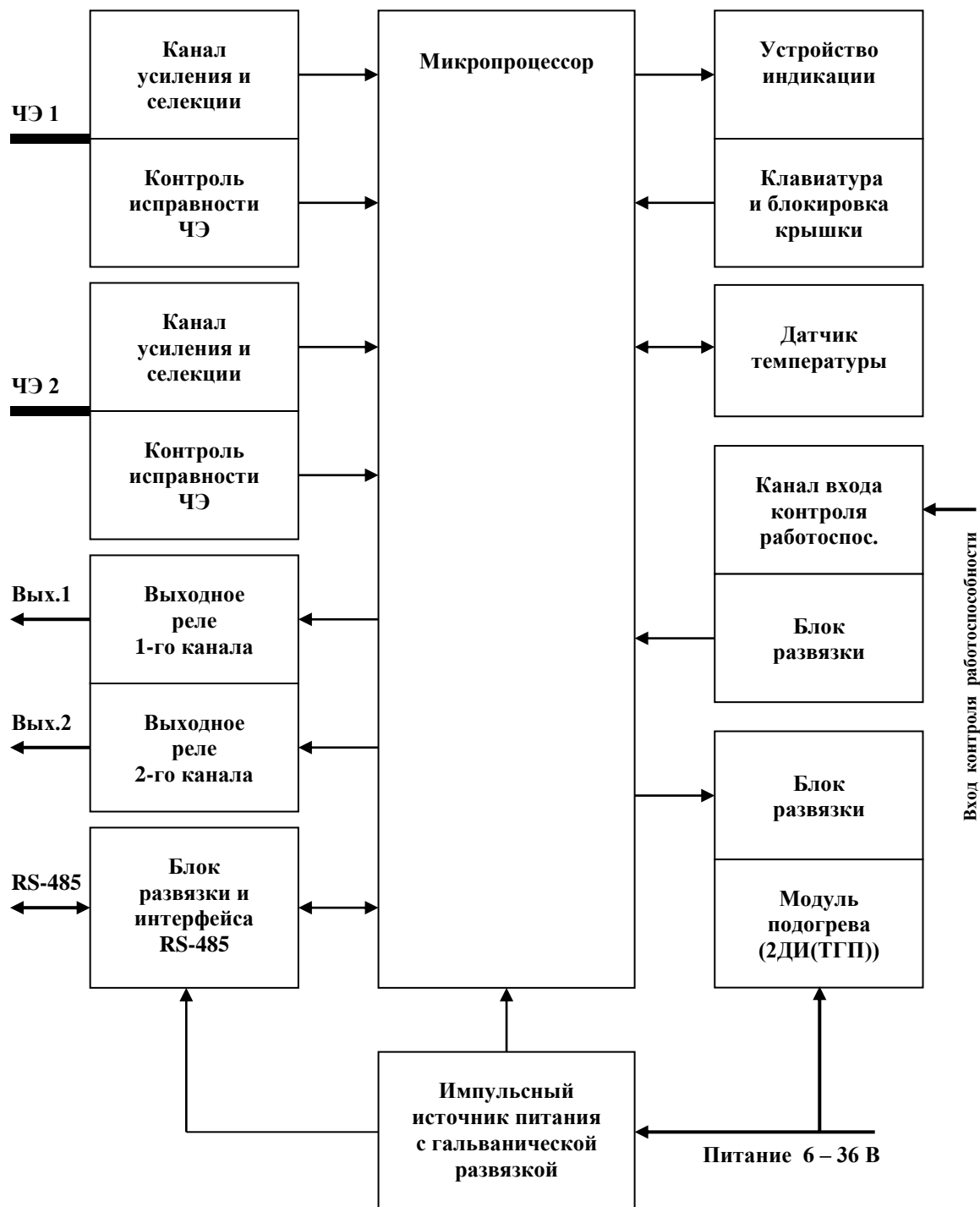
Рис. 9.1. Структурная схема изделия «Багульник-М»
