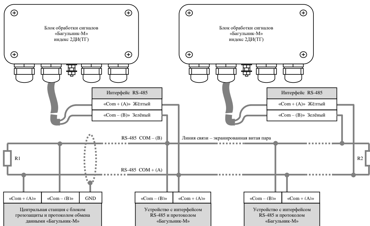
Рисунок 8.7. Подключение интерфейса RS-485 и организация линии связи
